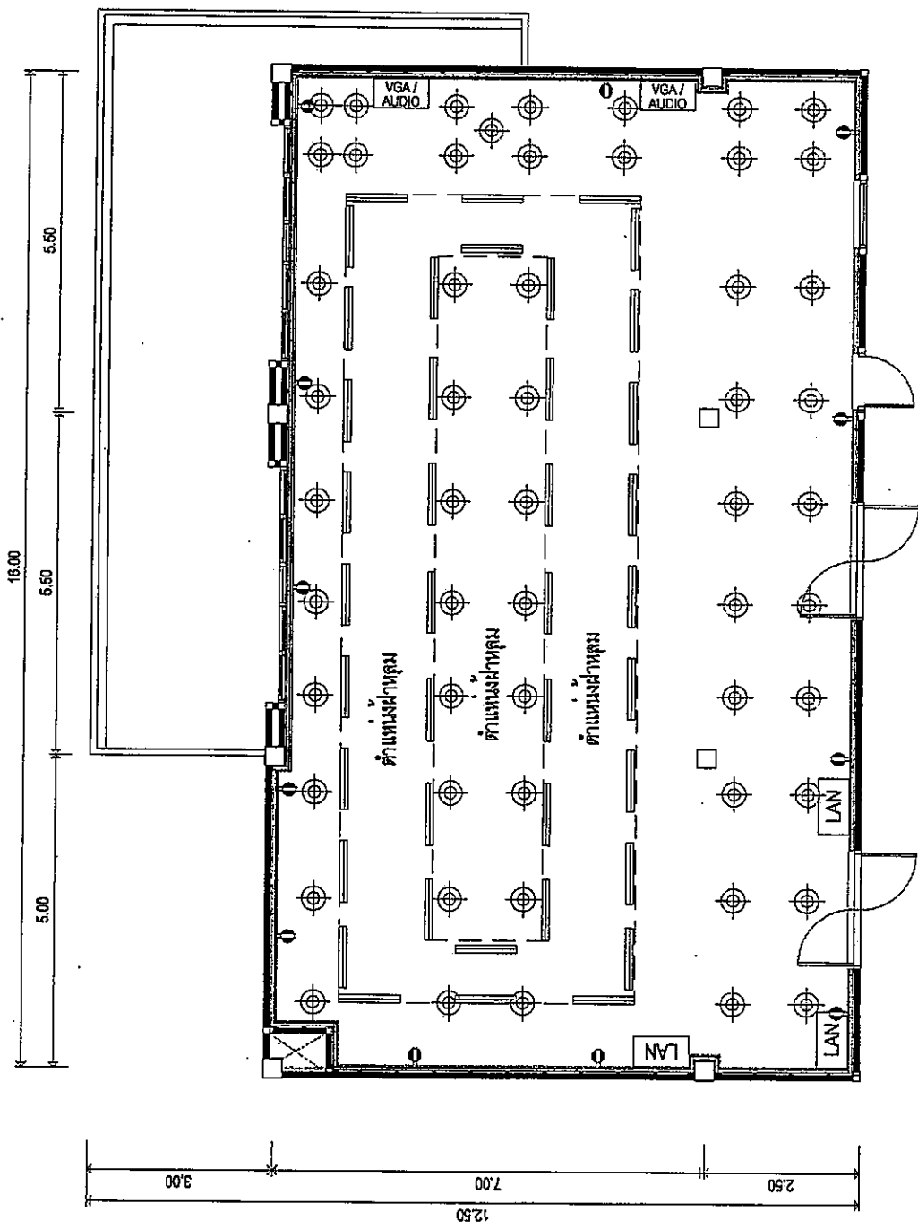
แปลนวางโต๊ะ, สวิตช์, ปลั๊กและฝังฝ้าเพดาน (เดิม) ขนาดตาม 1 : 50
